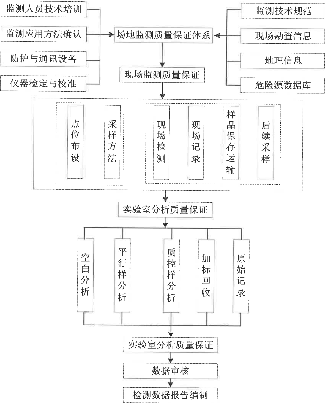
图 5.1-1 质量保证与质量控制体系
